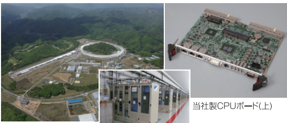
Spring8に完成したX線自由電子レーザー施設(SACLA)(左)のクライストロンギャラリー(下)加速管制御の心臓部を担う
